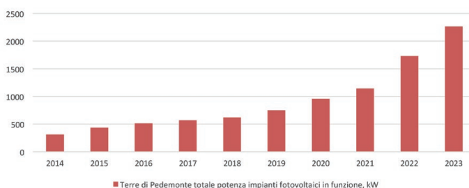
Terre di Pedemonte totale potenza impianti fotovoltaici in funzione, [kW]
